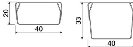
Metallkanal SX 40x20, 2m [515846] Metallkanal SX 40x33, 2m [515847]
