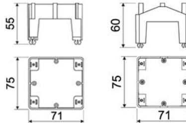
Insatsbox KP EKE [515830] Insatsbox KP PK [515831]
