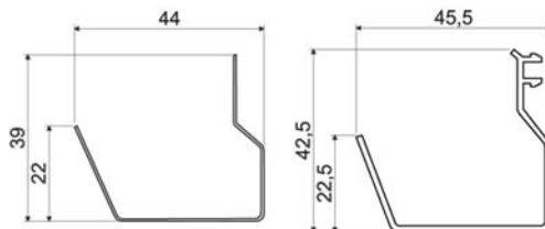
Kabelhållare PEP 60, 2m [515843] Kabelhållare metall PEP 60/K, 2m [515844]
