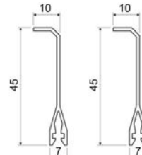
Avdelare PEKE 60, 2m [515841] Avdelare metallfolie PKS 70/60, 2m [515842]
