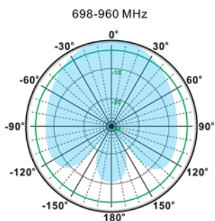
H-Plan
