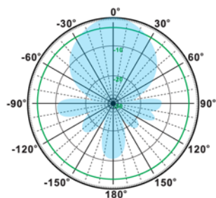
V-Plan
